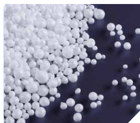
Corindons globulaires
