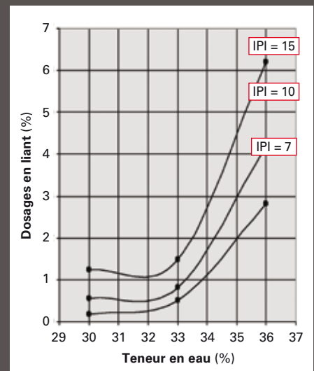
Dosages en liant nécessaires pour l'obtention d'un indice portant immédiat (IPI) de 7, 10 ou 15 en fonction des teneurs en eau
