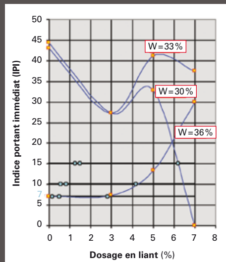
Évolution de l'indice portant immédiat (IPI) en fonction du dosage pour différentes teneurs en eau du sol
